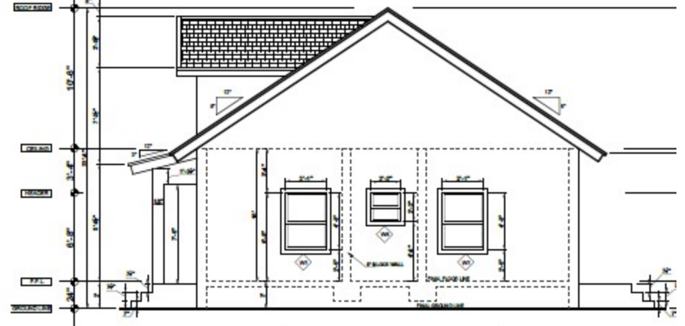
2 RIGHT ELEVATION SCALE: 1/4"=1'-0"
