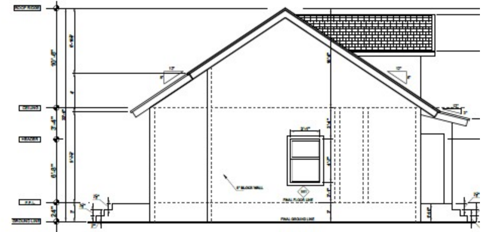
4 LEFT ELEVATION SCALE: 1/4"=1'-0"
